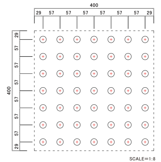
点字鋳基本配列(JIS)400角の場合 7×7 49個
