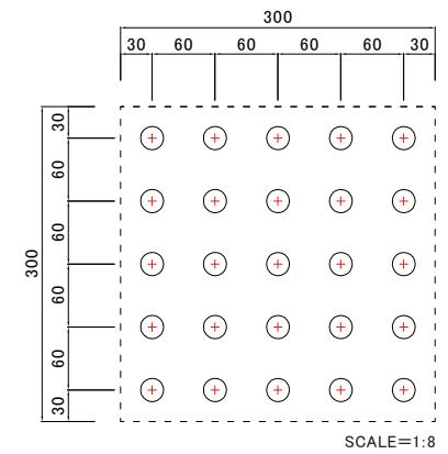
点字鋳基本配列(JIS)300角の場合 5×5 25個
