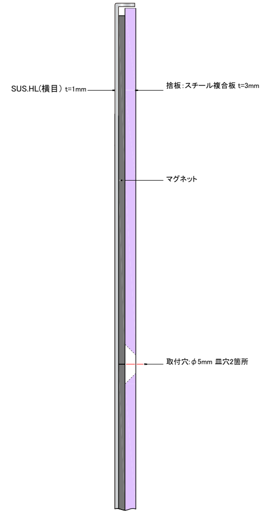
A-A SCALE 1:1
